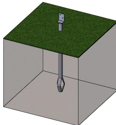
Efter installationen i marken expanderas nedre delen av Grundtuben med hjälp av expansionsverktyg.
